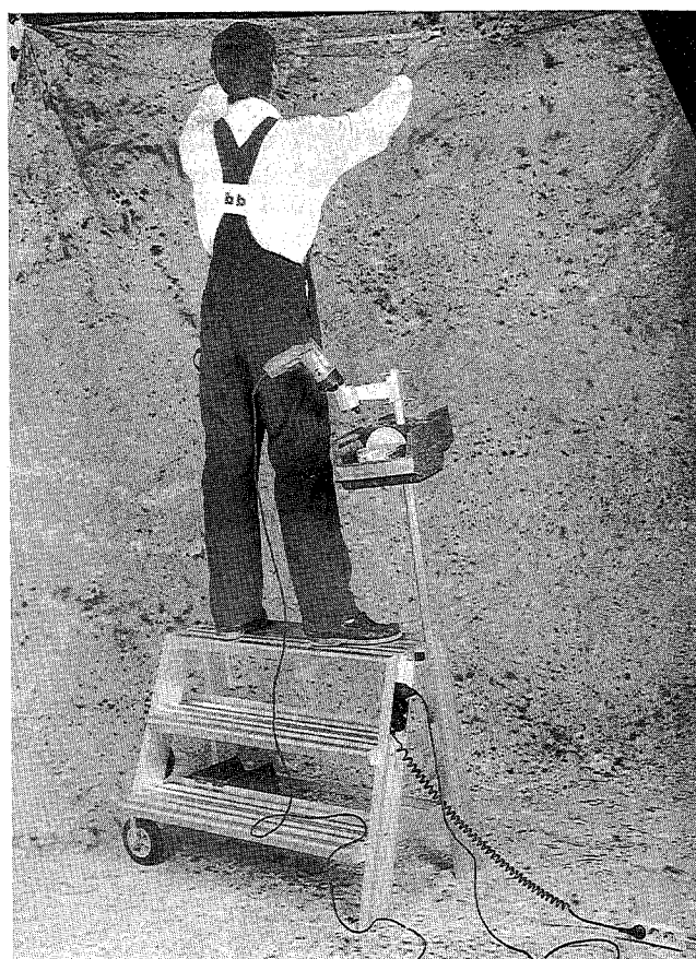
Fig 1 Verktyg och material i bekväm närhet för montören
