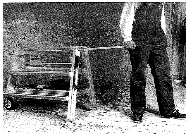
Fig 2 Utdragbart handtag för transport
